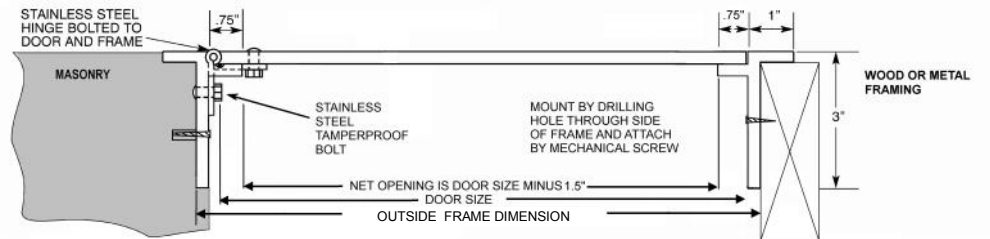
DOUBLE DOOR
