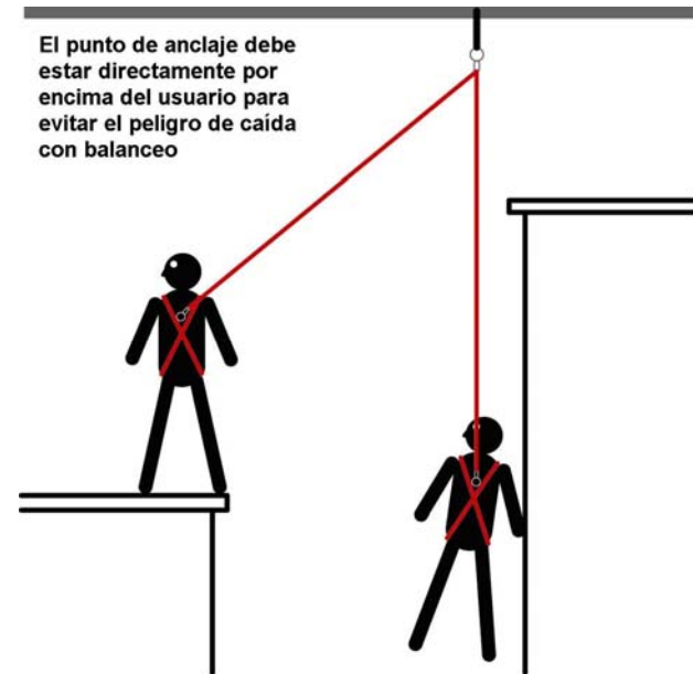
Figura 2.2: Diagrama de caída con balanceo
