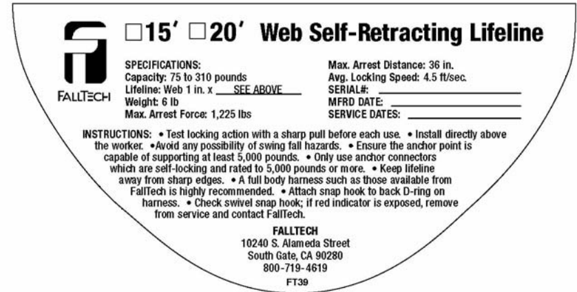
Fig. 10.2 Etiqueta del producto para las SRL de red de FallTech 7270WR, 7271WR y 7270KV (Situada en la cubierta delantera)
